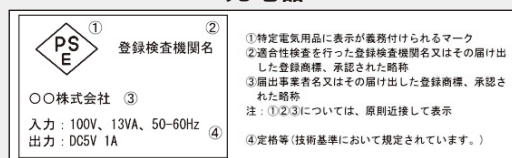
PSEマークの例(直流電源装置)
