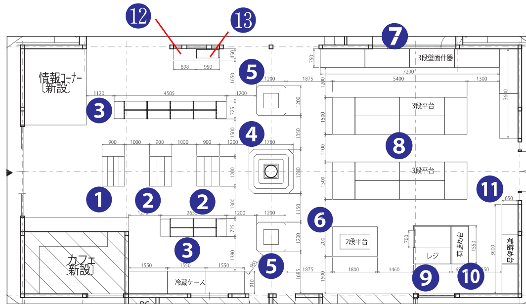
3 ■棚什器 KJ RACK APタイプ 島 各棚下LED付
