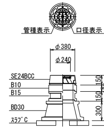
φ250 (土被り H=900)
