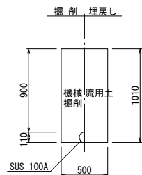
仮土工-2 (撤去)
