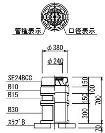
φ100 (土被り H=900)
