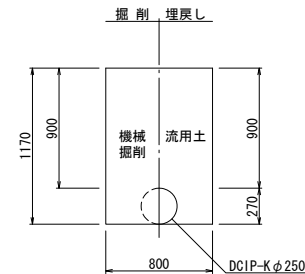
仮土工-6 (栓止工)
