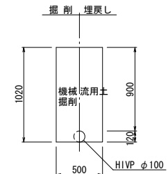
仮土工-7 (栓止工)
