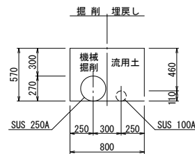
仮土工-3 (撤去)
