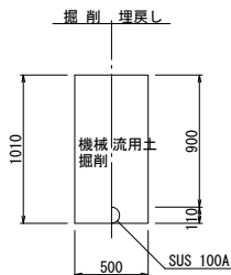
仮土工-2 (布設)
