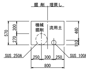
仮土工-3 (布設)
