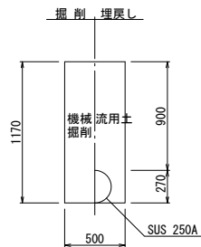
仮土工-1 (布設)
