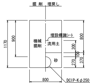
土工-1
