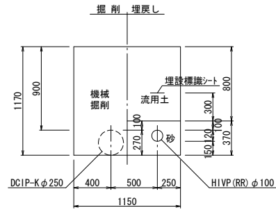
土工-3
