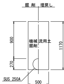
仮土工-1 (撤去)
