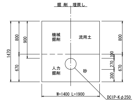
仮土工-5 (ストップ・バルブ)
