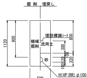
土工-2
