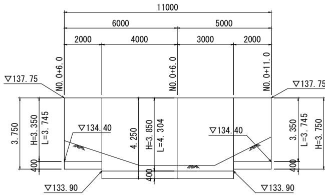
展開図 S=1:100
