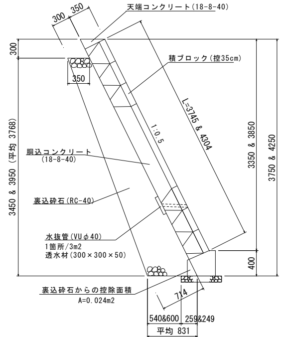
コンクリートブロック積工 構造図 S=1:30
