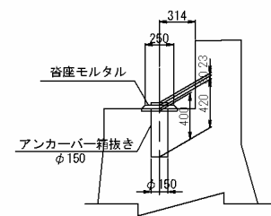
断面図 S=1:25
