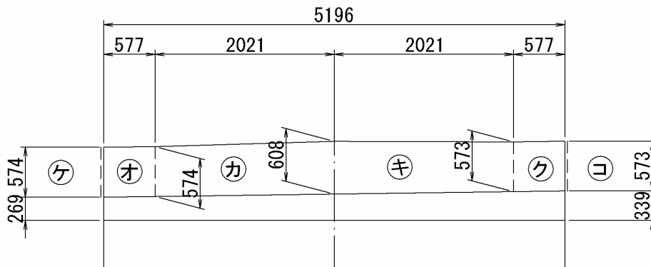
背面図
