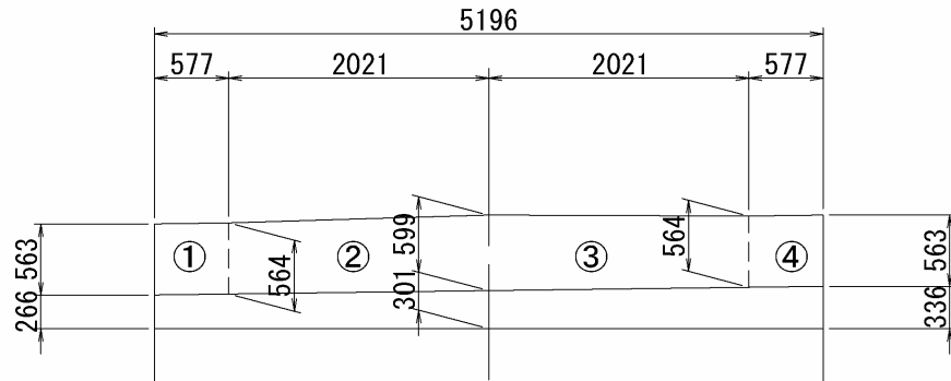
正面図
