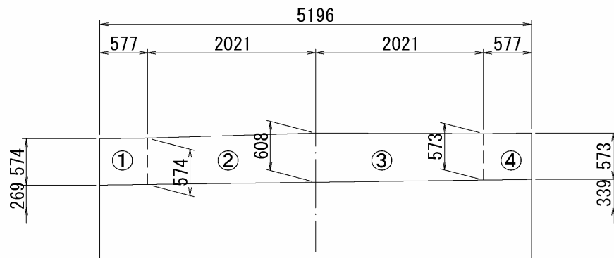
背面図
