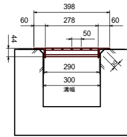
現場打ち側溝 (B300 : 面取) N=10枚 (普通目 : T-14)
