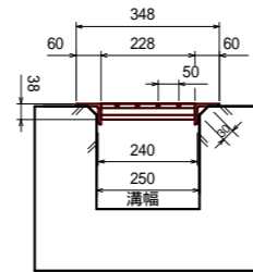
現場打ち側溝 (B250 : 面取) N=116枚 (普通目 : T-14)
