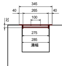
現場打ち側溝 (B285) N=3枚 (細目 : T-14)
