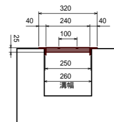
現場打ち側溝 (B260) N=6枚 (細目 : T-14)
