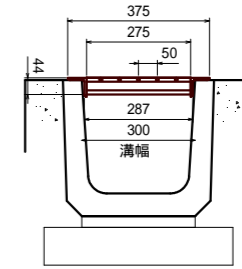
鉄筋コンクリート側溝 PU300 N=6枚 (普通目 : T-14)
