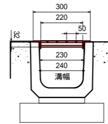
鉄筋コンクリート側溝 PU240 N=95枚 (普通目 : T-14)
