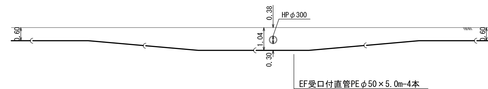
c-c' 断面图 S=1/100 C09+1.27
