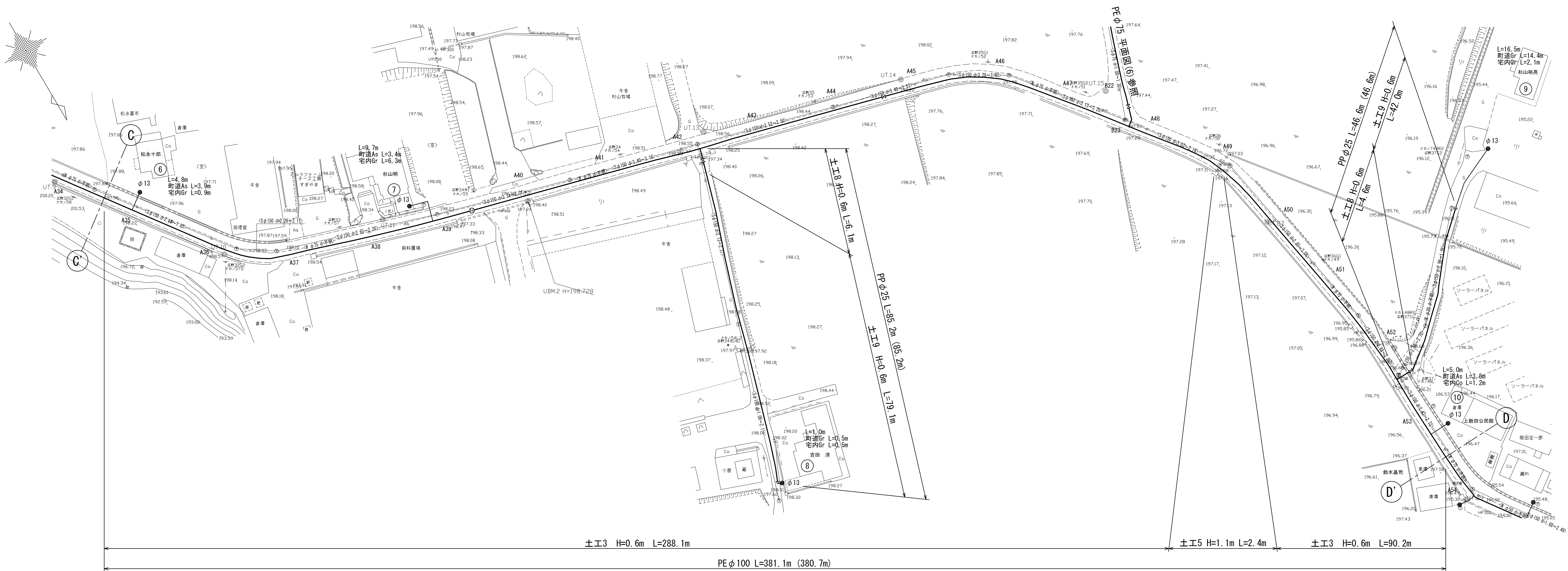
平面図(3) S=1/500
