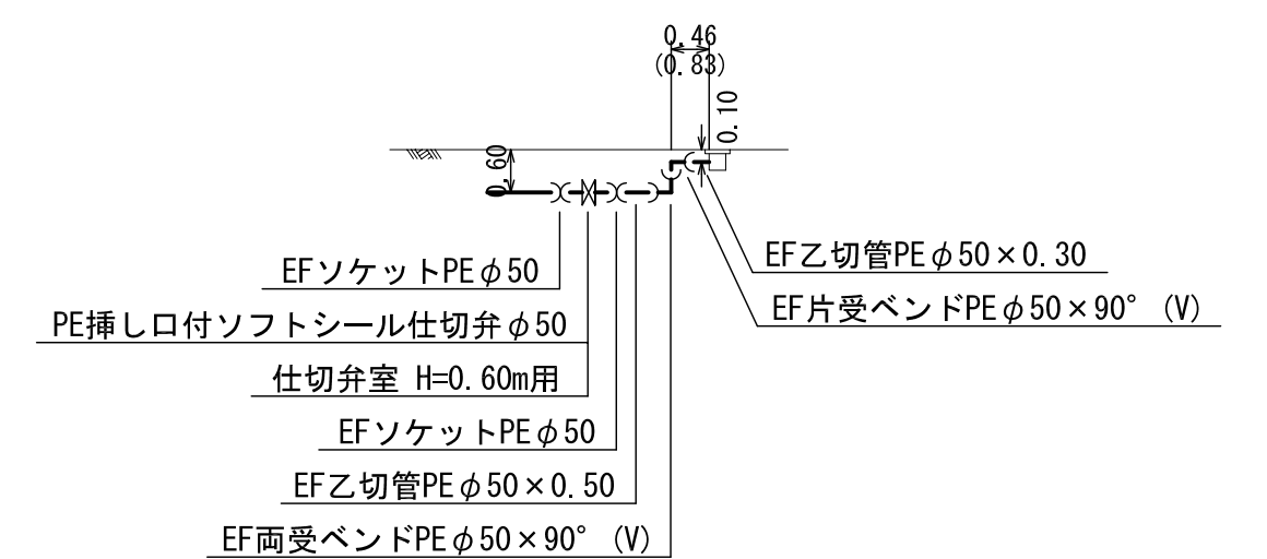
d-d' 断面图 S=1/100
