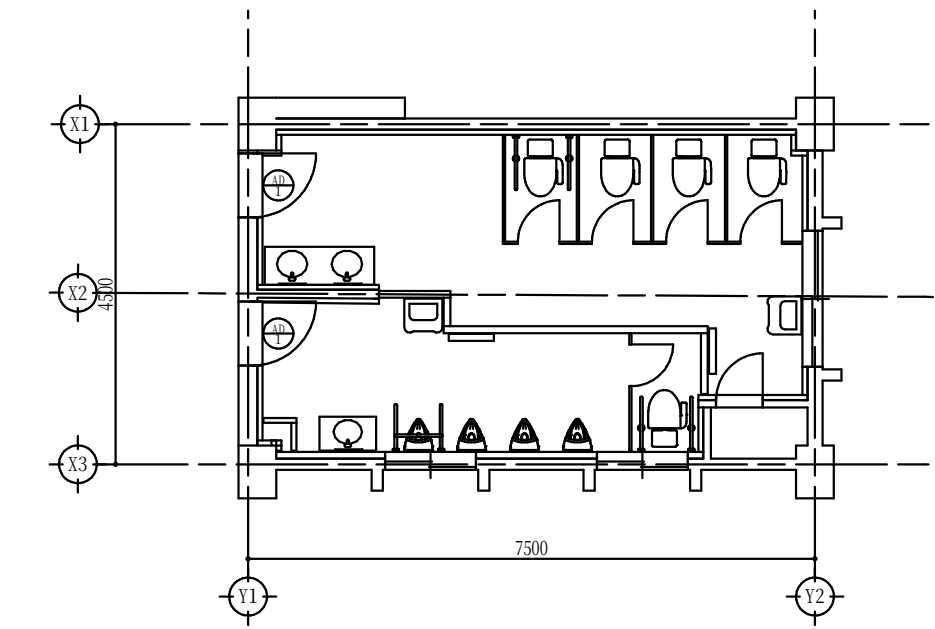
男子・女子生徒便所（1～3階まで共通）建具配置図 1/100
