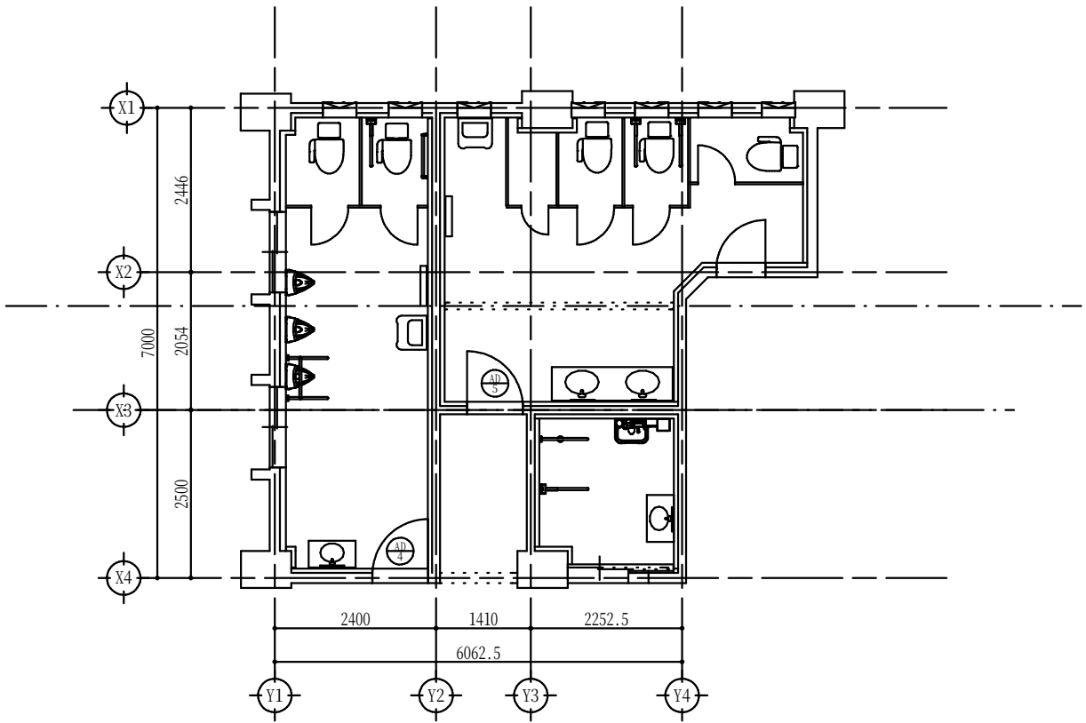
男子・女子生徒・多目的トイレ（1階）建具配置図1/100
