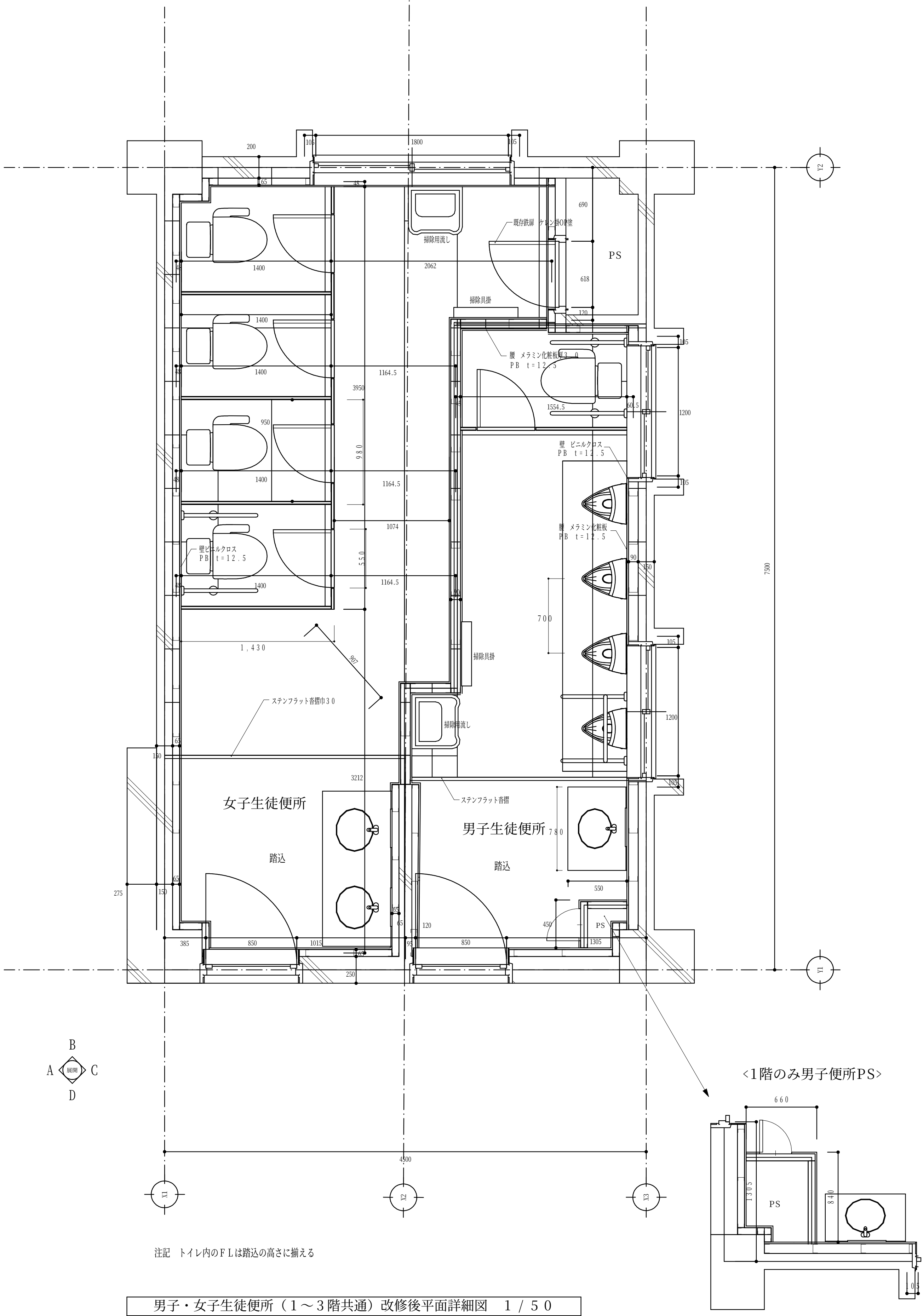
男子・女子生徒便所（1～3階共通）改修後平面詳細図 1 / 5 0
