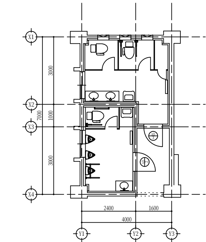
男子・女子職員便所（2階）建具配置図1/100
