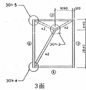
3面
