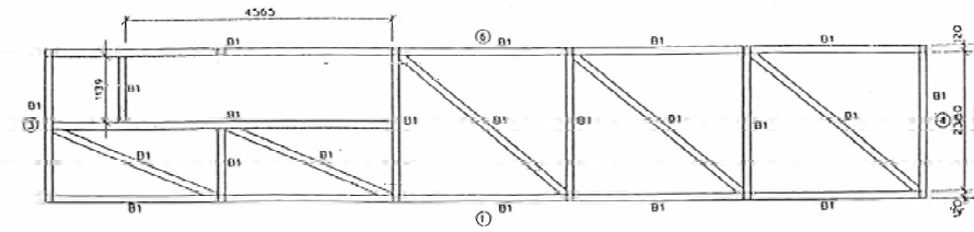
上部 (2面)
