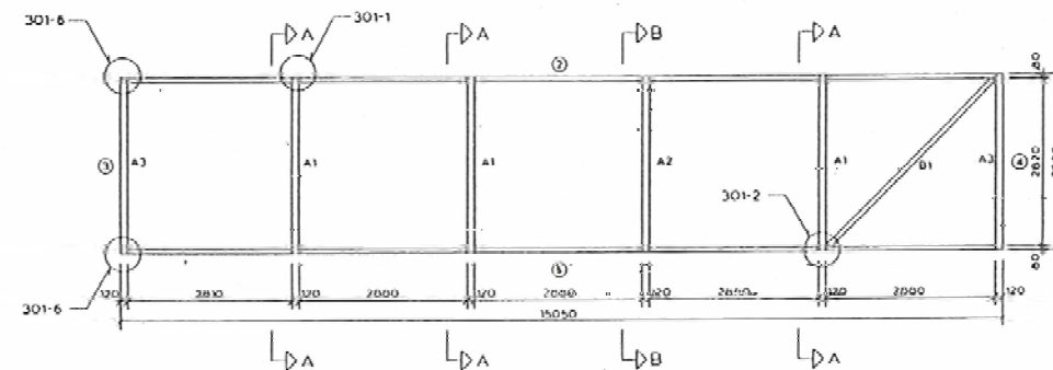
前部 (1面)
