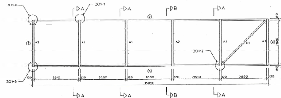
前部 (1面)
