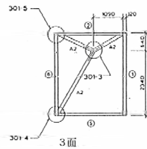
3面
