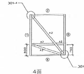
4面
