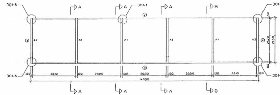
前部 (1面)
