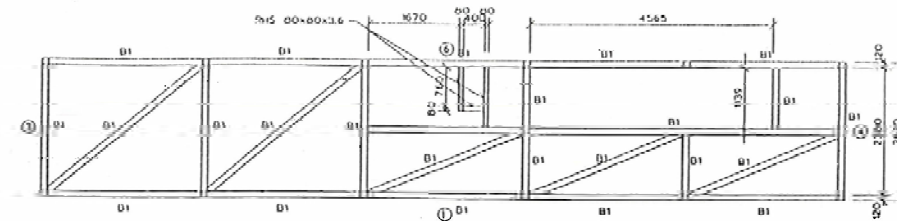
上部 (2面)
