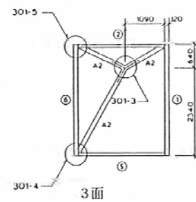
3面
