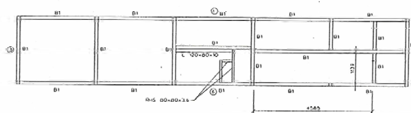
下部 (5面)
