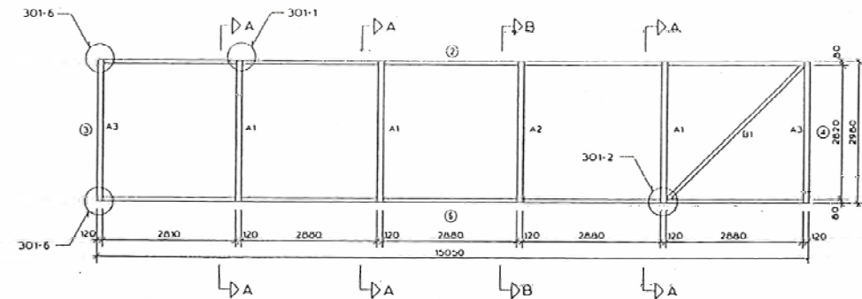
前部 (1面)
